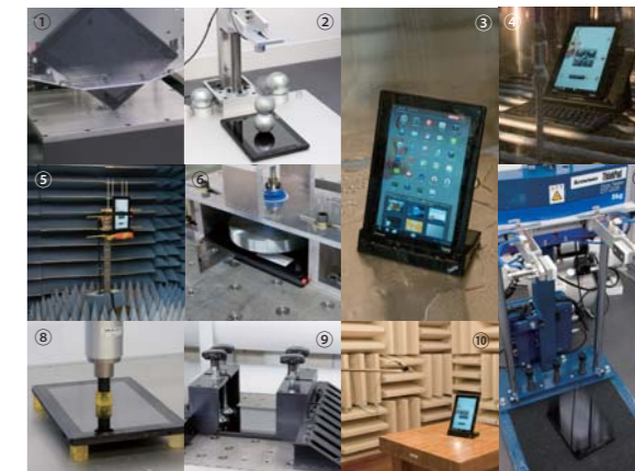
①角落下試験 ②液晶面鉄球落下試験 ③防滴試験 ④防塵試験 ⑤無線性能試験 ⑥加圧振動試験 ⑦自由落下試験 ⑧LCDストレステスト ⑨反復繰り返し衝撃試験 ⑩動作ノイズ測定試験
