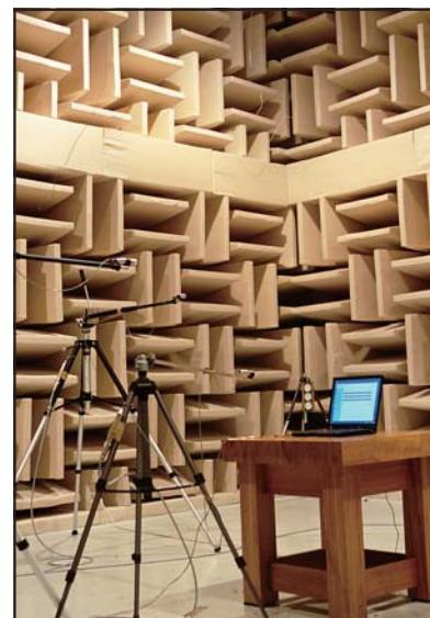
⑩動作ノイズ測定試験 音響測定用の専用の部屋でThinkPadの出す音を測定する。
