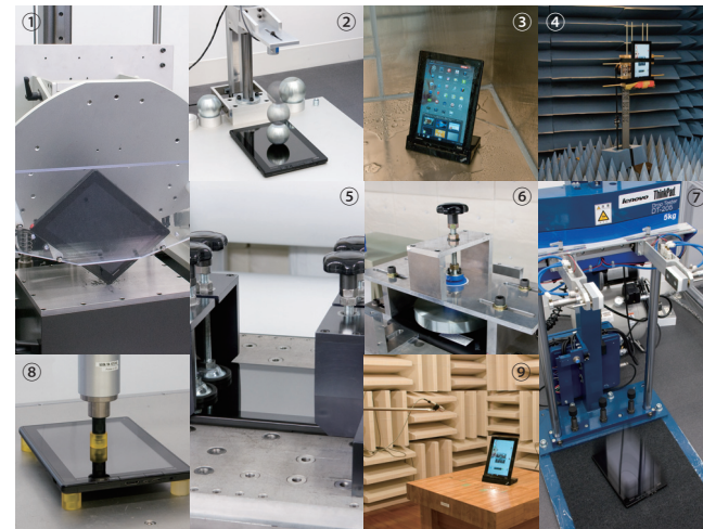
①角落下試験 ②液晶面鉄球落下試験 ③防滴試験 ④無線性能試験 ⑤反復繰り返し衝撃試験 ⑥加圧振動試験 ⑦自由落下試験 ⑧LCDストレステスト ⑨動作ノイズ測定試験
