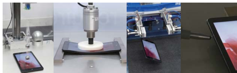
液晶面鉄球落下試験 LCDストレステスト 自由落下試験 静電気耐性試験
