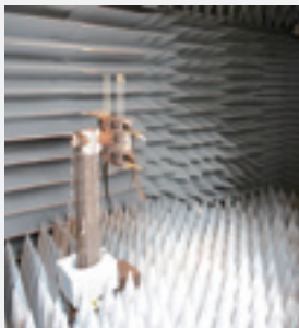
無線性能試験
