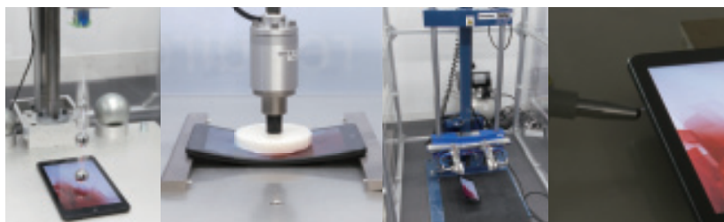
液晶面鉄球落下試験
