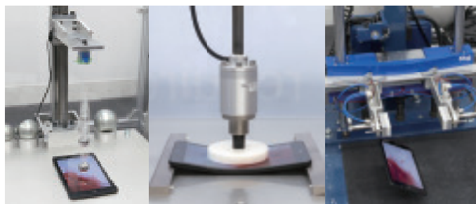
液晶面鉄球落下試験
