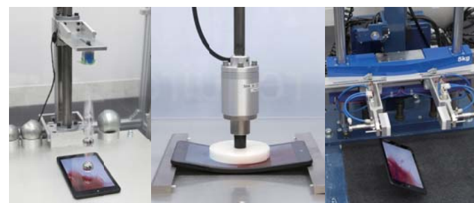
液晶面鉄球落下試験 LCDストレステスト 自由落下試験
